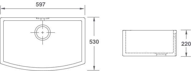
W:597 x D:530 x H:220mm
