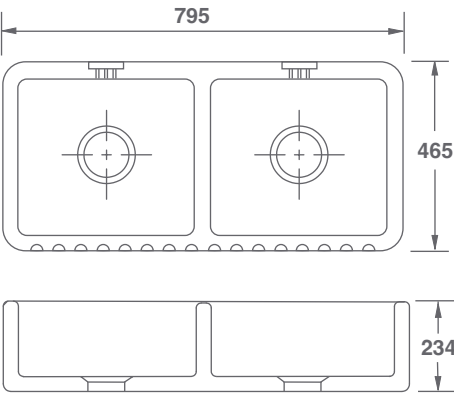
W:795 x D:465 x H:234mm
