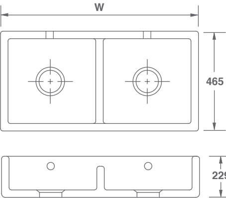
800 – W:795 x D:465 x H:229mm
